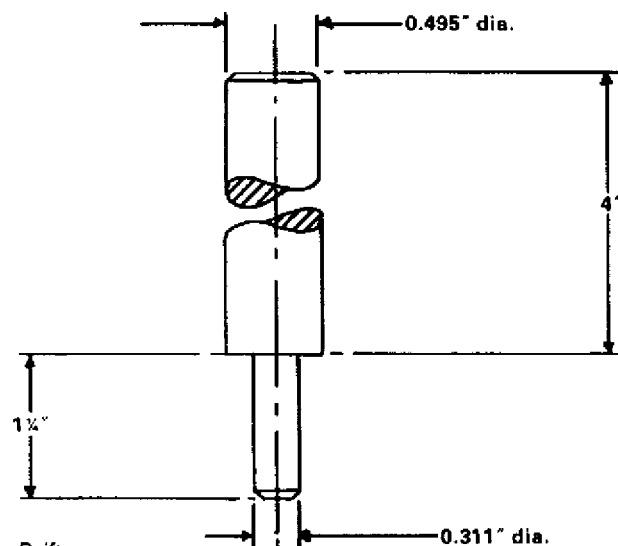
Fig. 13. Drift.
